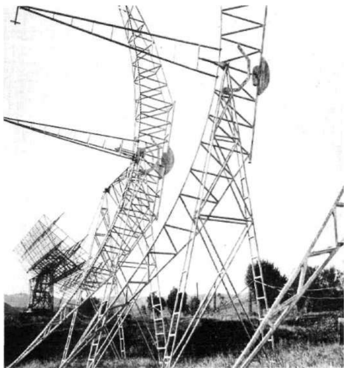
Část anténního systému pro odposlech signálů ze vzdálenosti mnoha světelných let, instalovaného ve stanici Gor- ký.
